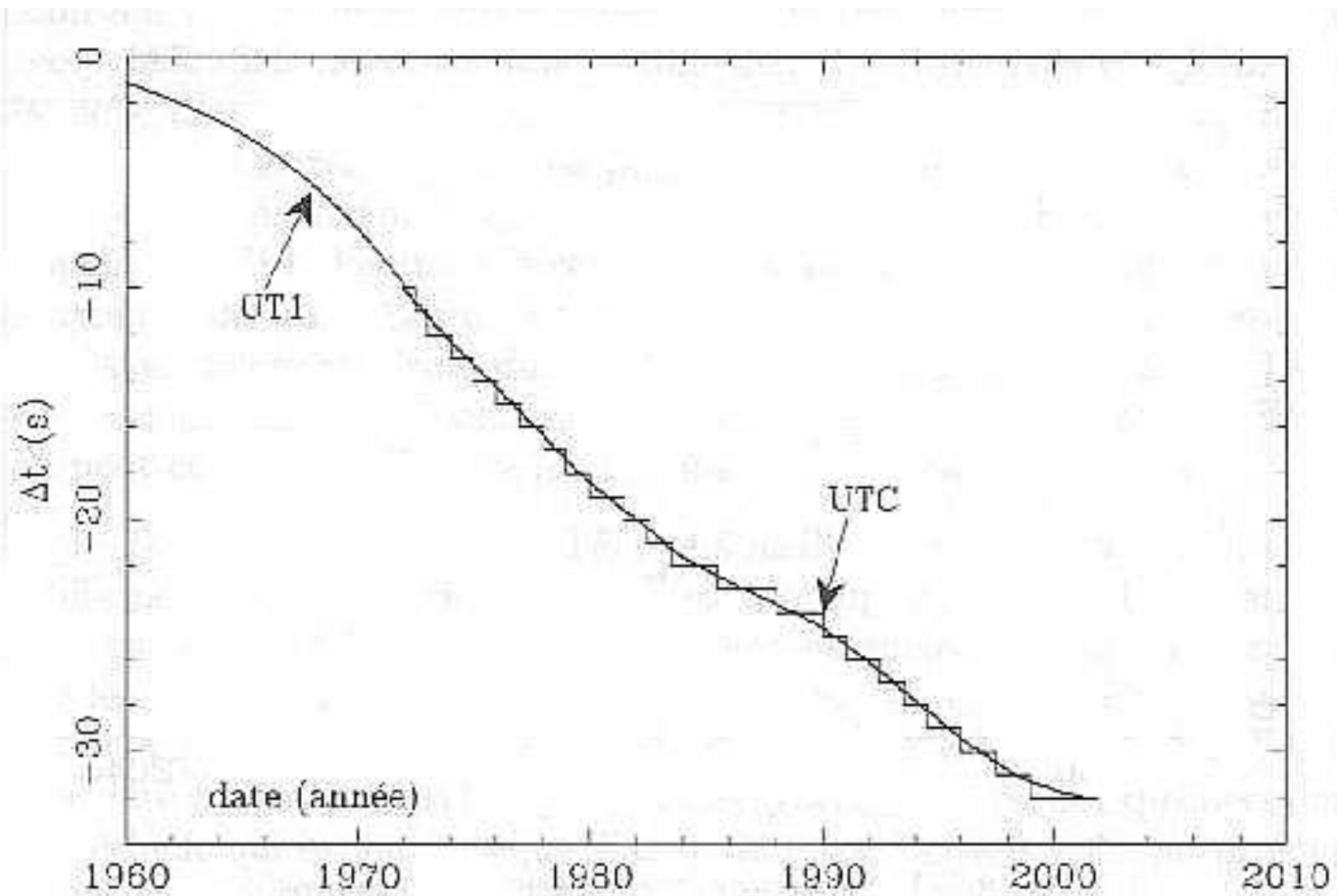
Différences en secondes par rapport au TAI.
